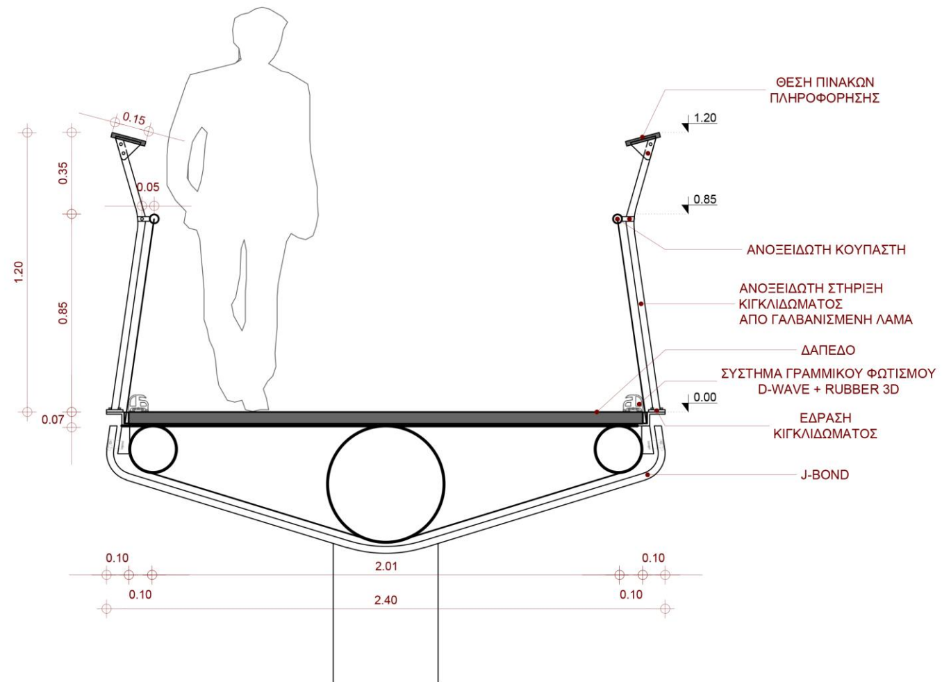
ΛΕΠΤΟΜΕΡΕΙΑ ΚΙΓΚΛΙΔΩΜΑΤΟΣ ΣΕ ΠΑΣΑΡΕΛΑ ΚΑΙ ΠΛΕΥΡΙΚΟΥΣ ΕΞΩΣΤΕΣ
